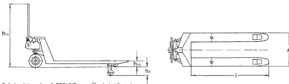
Ručný paletovací vozík PROLINE s predĺženými vidlicami Ručný paletovací vozík PROLINE s predĺženými vidlicami a zvýšenou nosnosťou
