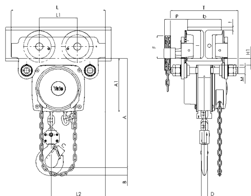
Model Yalelift ITG, 500 - 3000kg, jednoramenný
