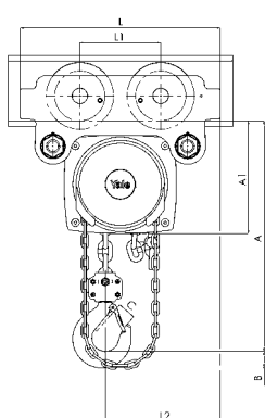
Model Yalelift ITP, 500 - 3000kg, jednoramenný
