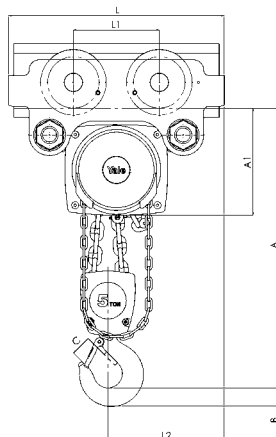
Model Yalelift ITP/ITG, 5000kg, dvojrarmenný
