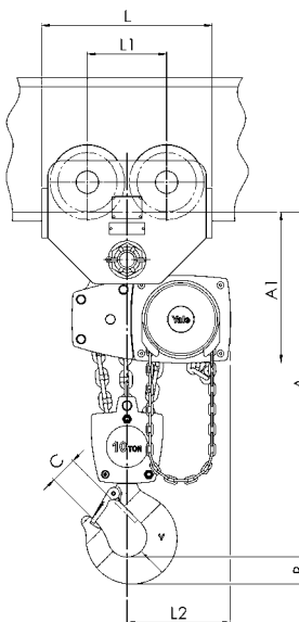
Model Yalelift ITG, 10000kg, trojramenný
